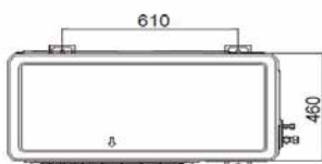
Yksikön mitat, mallit IGZAW12SNO3-1, IGZAW14SNO3-1, IGZAW14SNO3-1
