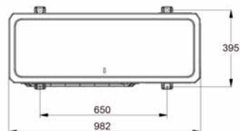
Yksikön mitat mallit IGZAW8SNO-1, IGZAW10SNO-1, IGZAW8SNO3-1, IGZAW10SNO3-1
