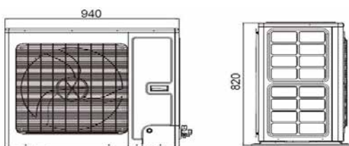
Yksikön mitat, mallit IGZAW12SNO3-1, IGZAW14SNO3-1, IGZAW14SNO3-1
